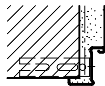
Maueranker montage
