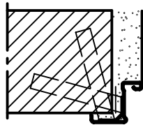
Maueranker montage nach DIN 18093
