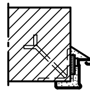
Anschweißmontage
