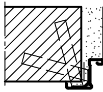
Mauerankermontage nach DIN 18093
