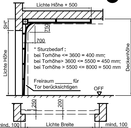
Normal-Beschlag
