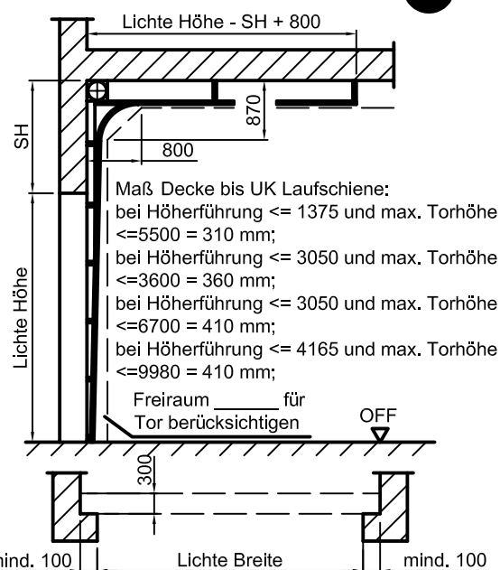
Höhergeführte-Laufschienen-Beschlag
