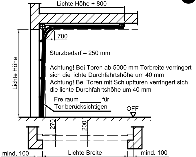
Niedrigsturz-Beschlag
